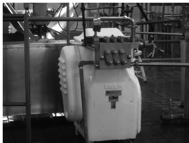
Figura 12 y 13 Efecto de la homogenización en los glóbulos grasos 7 y Equipo Homogenizador
