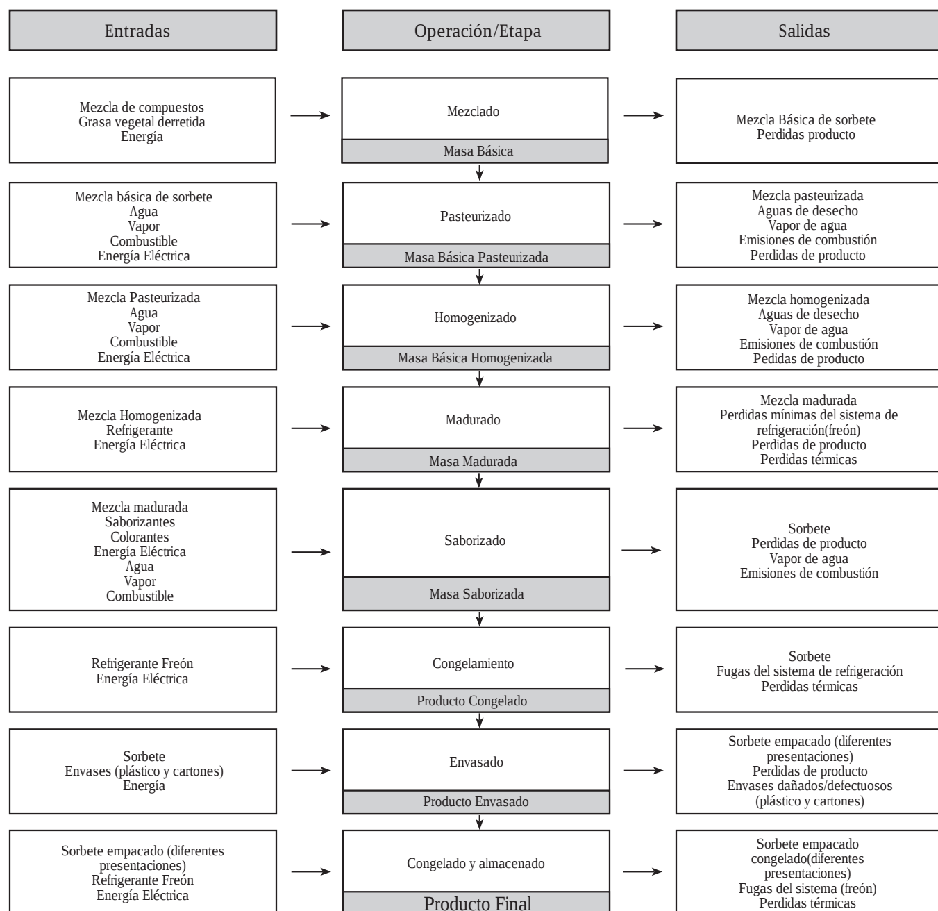
Figura 19 Diagrama de elaboración Helados
