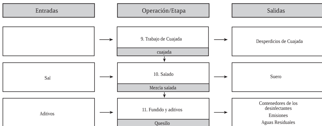
Figura 17. Diagrama de elaboración quesillo
