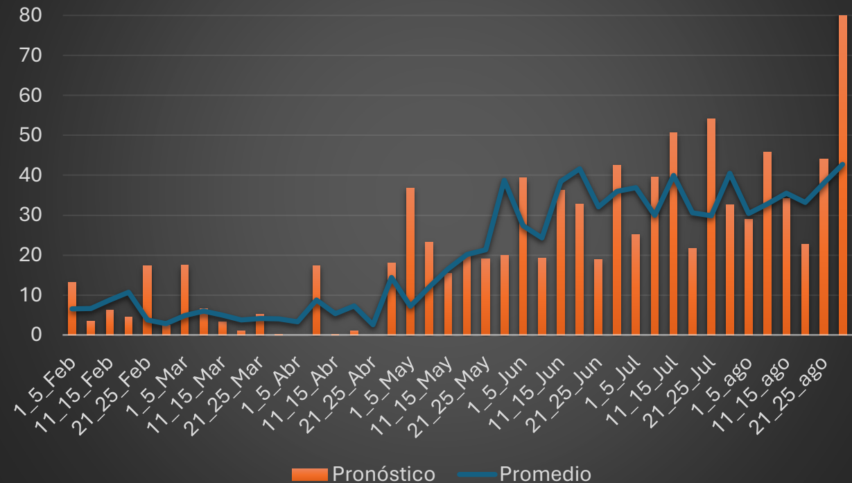
Pronóstico de lluvia, cada 5 días, Galeras, S. Bárbara, 2026
