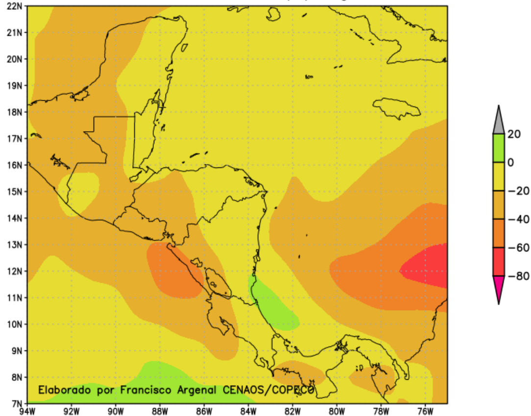
"Pronostico de anomalia de lluvia (%), Agosto 2026 NMME"
