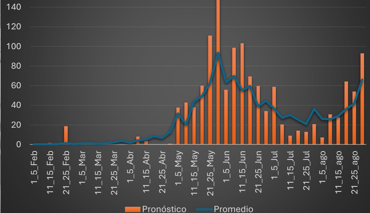
Pronóstico de lluvia, cada 5 días, Amapala 2026
