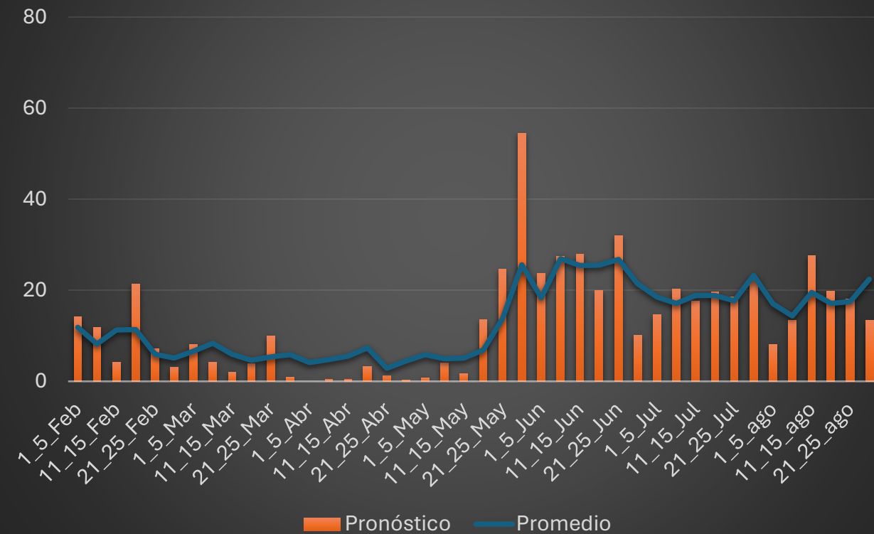
Pronóstico de lluvias en La Lima, 2026
