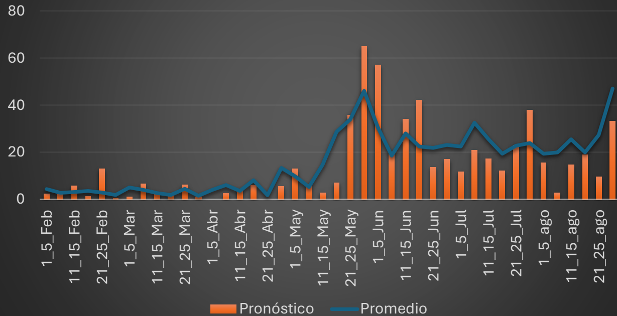
Pronóstico de lluvias en Lepaguare, cada 5 días, 2026
