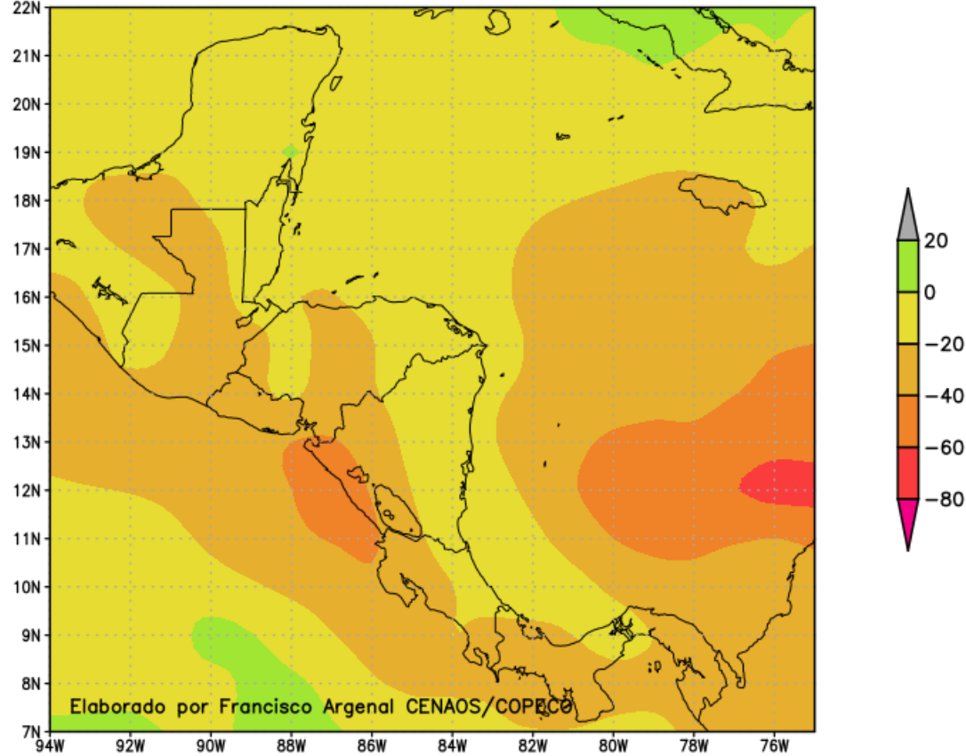
"Pronostico de anomalia de lluvia (%), Julio 2026 NMME"
