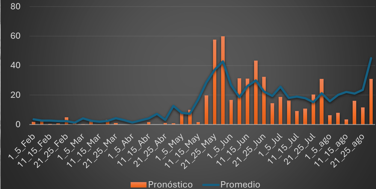
Pronóstico de lluvia, cada 5 días, Jacaleapa 2026
