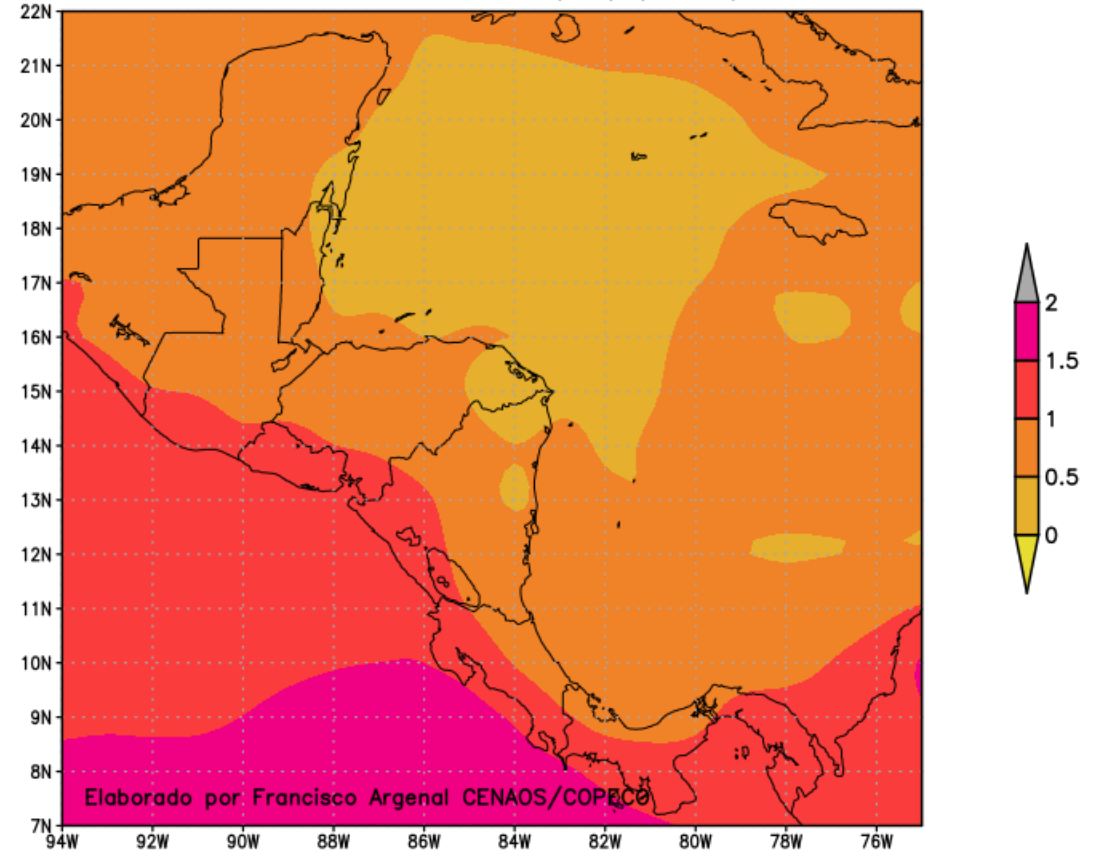
"Pronostico de anomalia de temp (C), septiembre, NMME"
