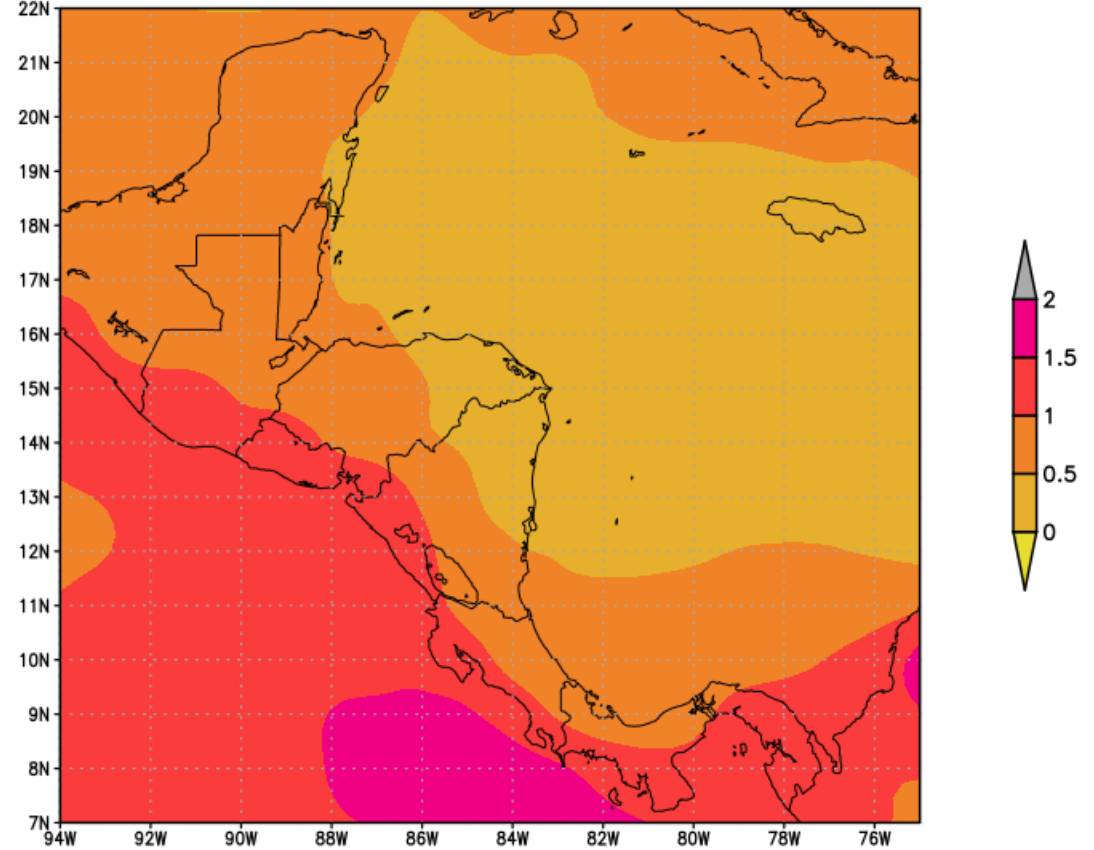
"Pronostico de anomalia de temp (C), Julio, NMME"
