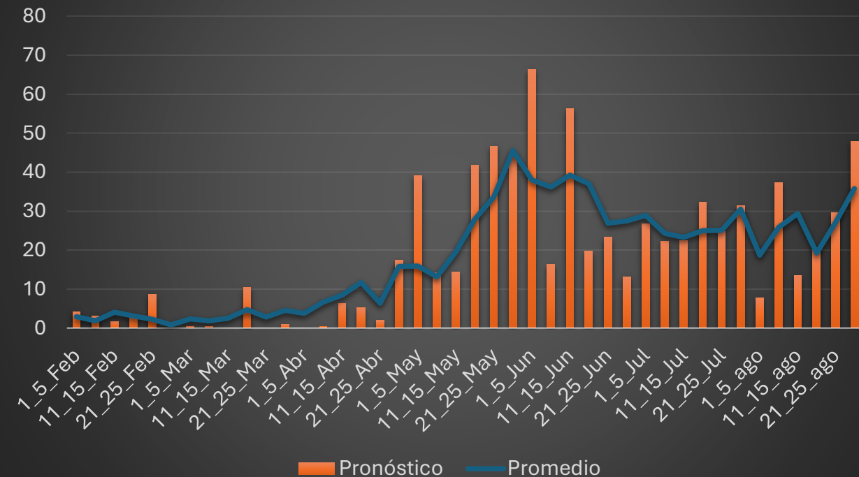
Pronóstico de lluvias, cada 5 días, Agua Caliente, FM, 2026
