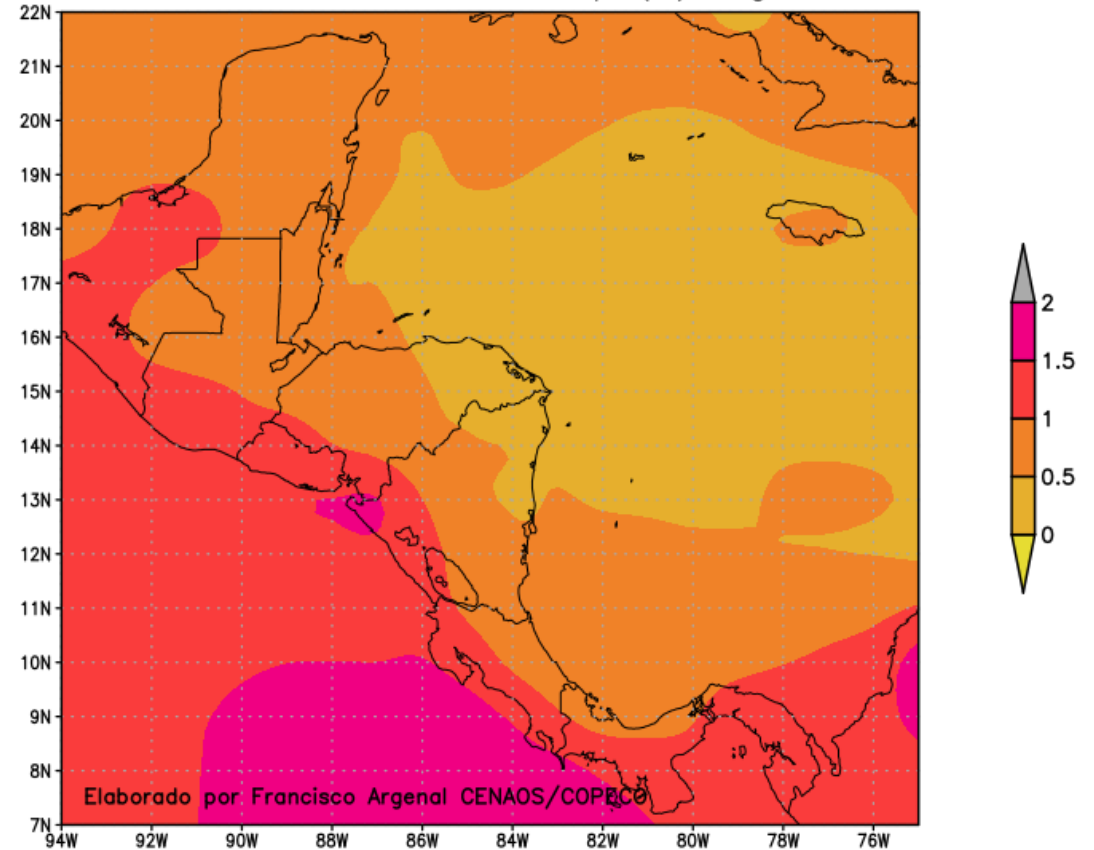
"Pronostico de anomalia de temp (C), agosto, NMME"
