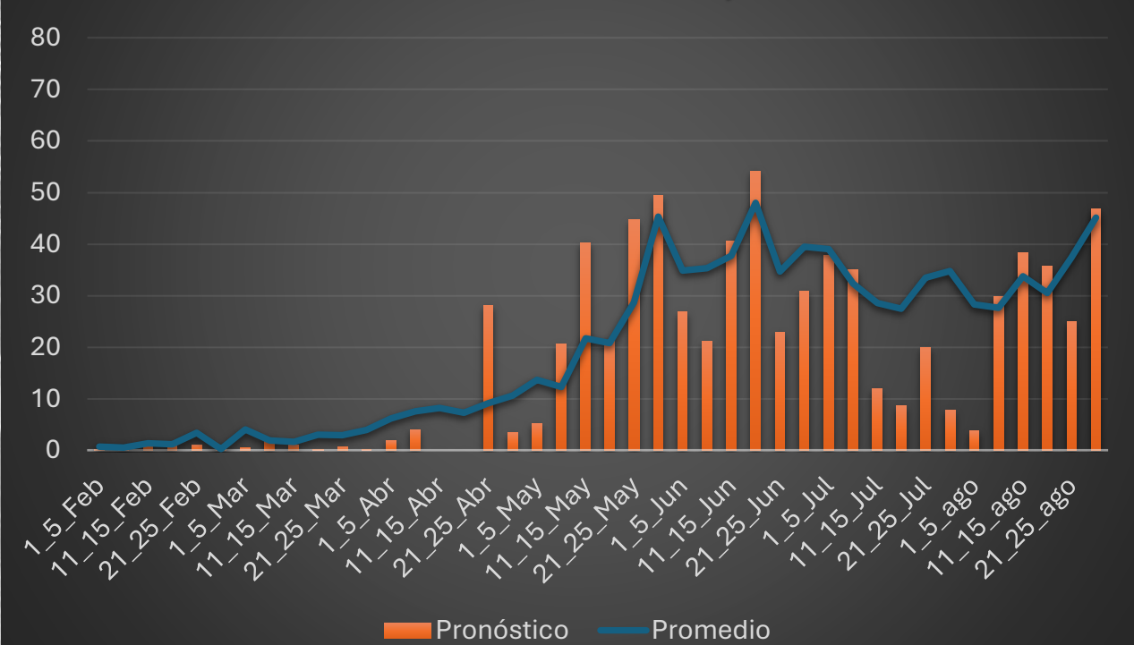
Pronóstico de lluvia, cada 5 días en La Labor, 2024
