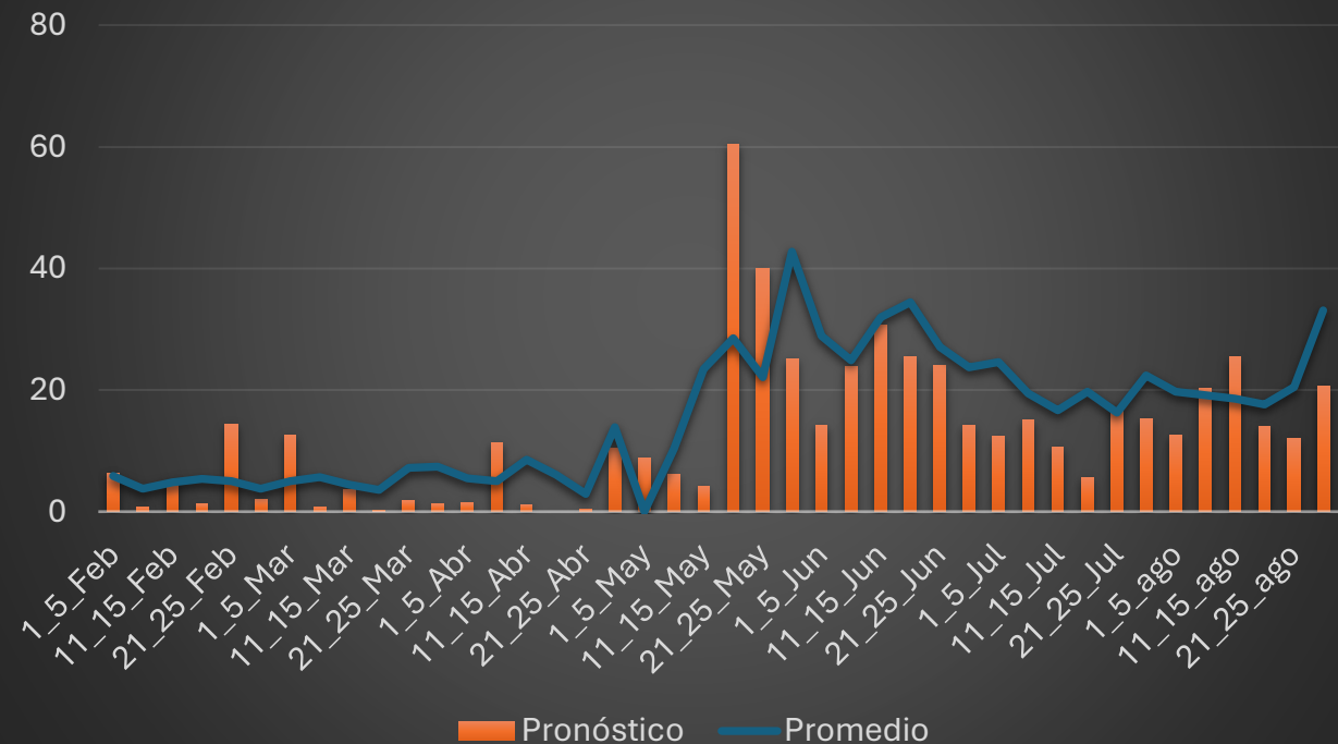
Pronóstico de lluvias, cada 5 días, Yoro, 2026
