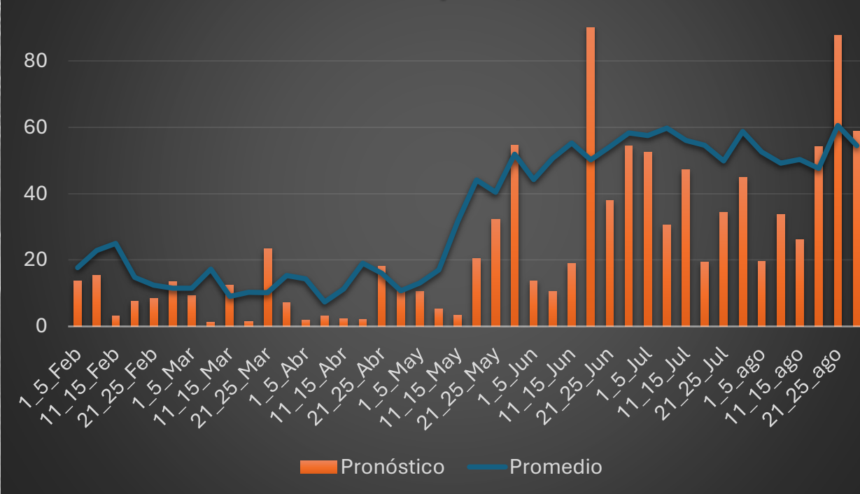
Pronóstico de lluvias, cada 5 días, Pto. Lempira, 2026
