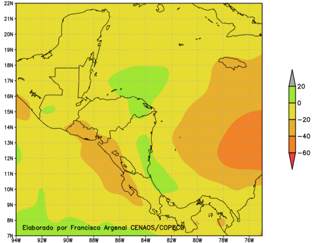
"Pronostico de anomalia de lluvia (%), Sept. 2026 NMME"
