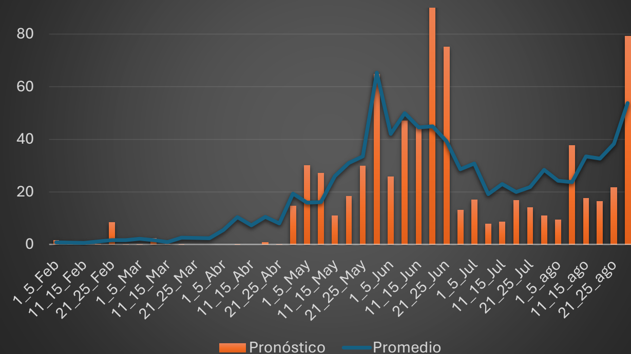
Pronóstico de lluvias, cada 5 días, La Esperanza, 2026
