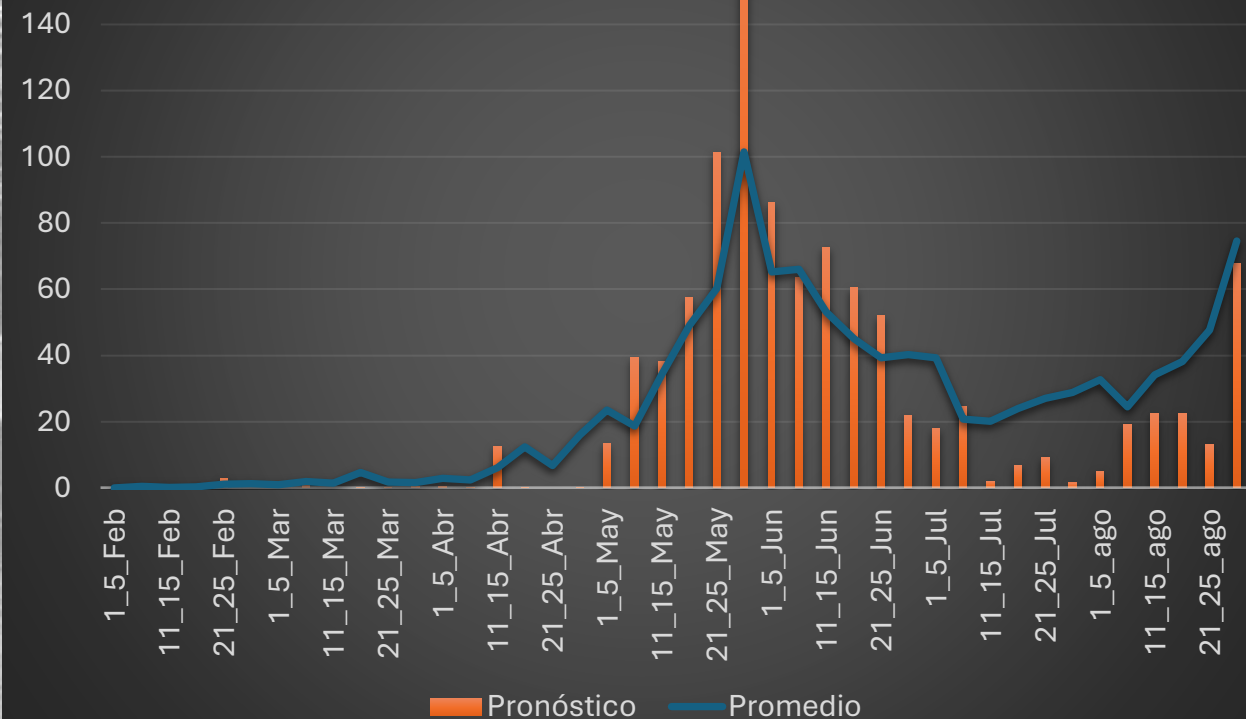
Pronóstico de lluvia en Choluteca, cada 5 días, 2026
