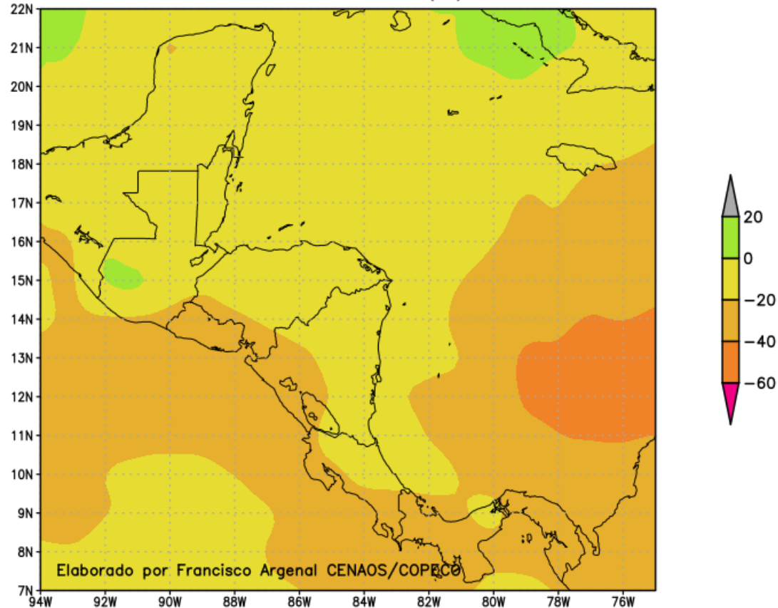
"Pronostico de anomalia de lluvia (%), Junio 2026 NMME"
