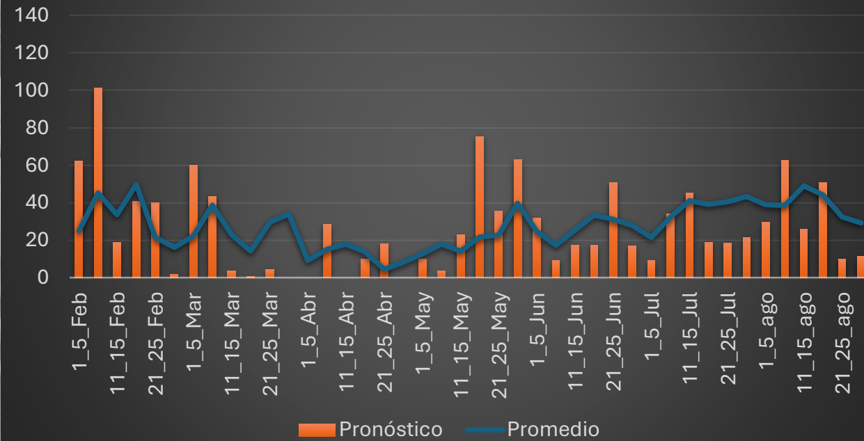
Pronóstico de lluvias en Omoa, cada 5 días, 2026
