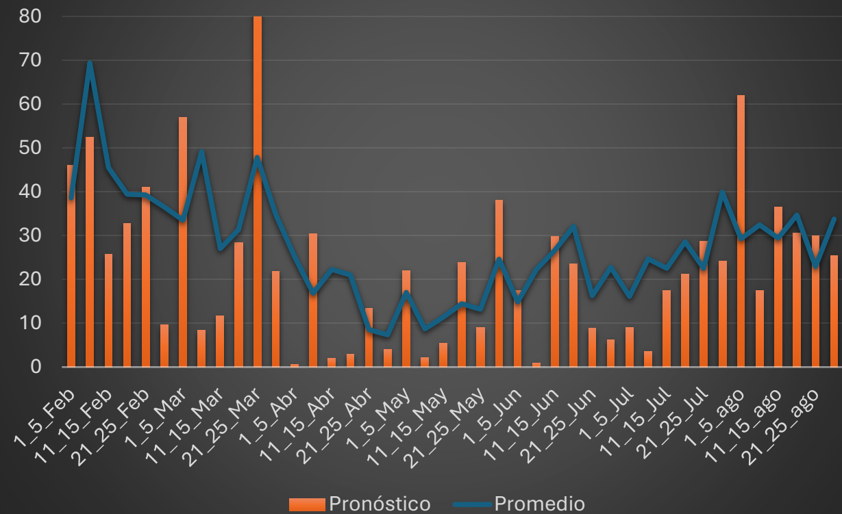
Pronóstico de lluvias, cada 5 días, La Ceiba, 2026
