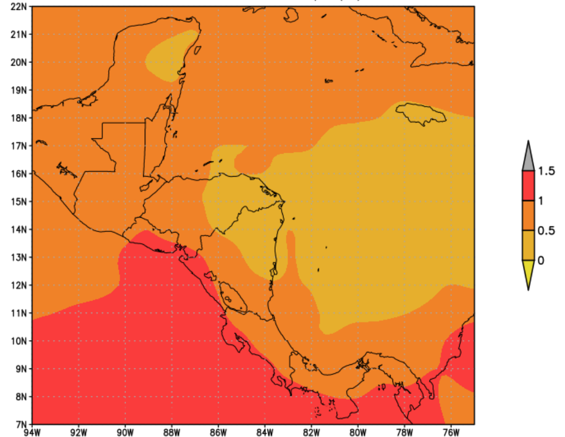
"Pronostico de anomalia de temp (C), Junio, NMME"
