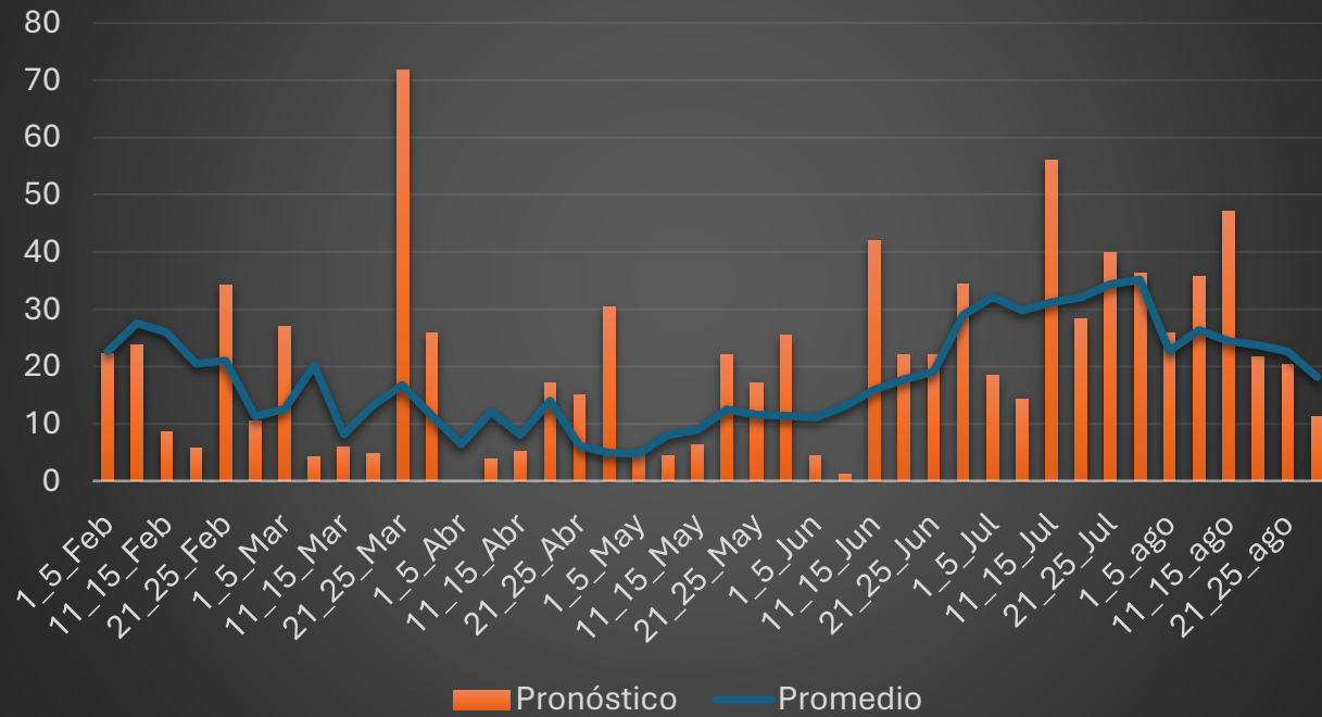
Pronóstico de lluvia, cada 5 días, Roatán, 2026
