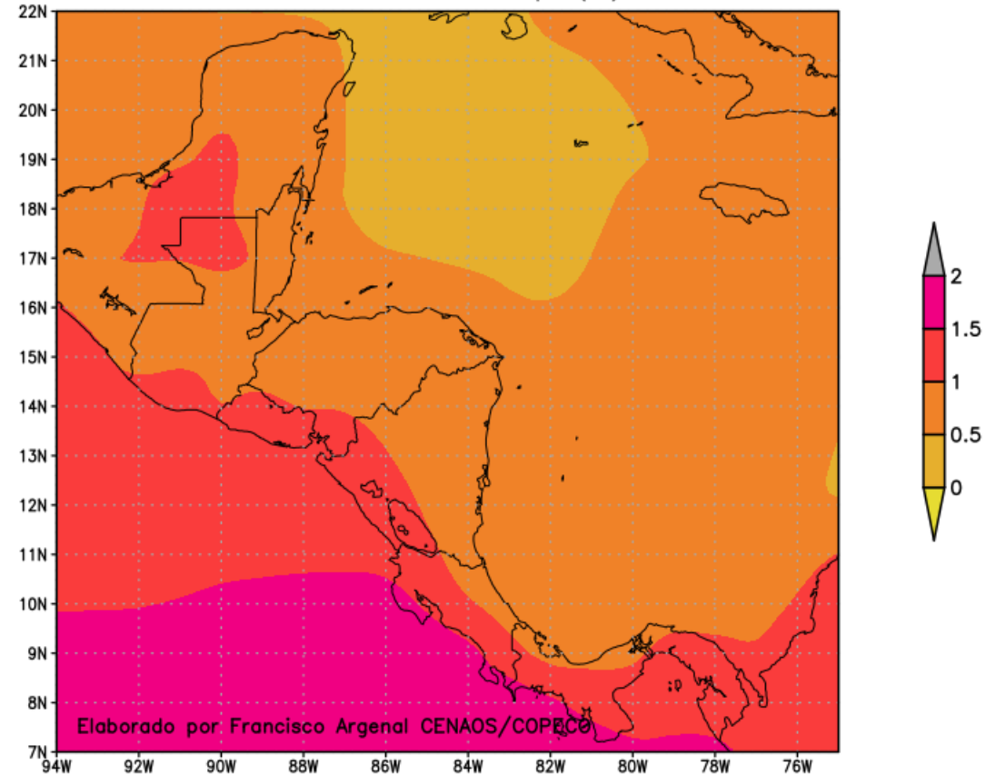
"Pronostico de anomalia de temp (C), octubre, NMME"
