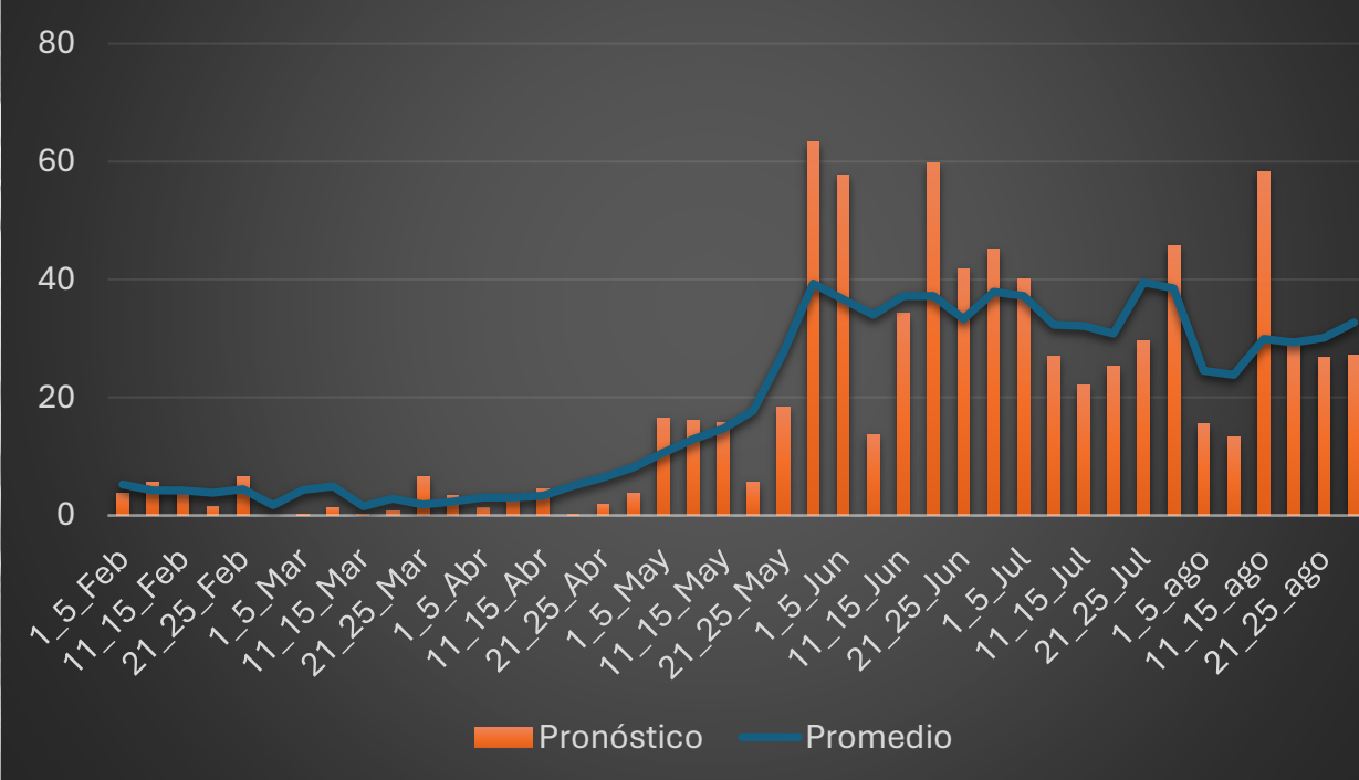
Pronóstico de lluvias, cada 5 días, Catacamas, 2026
