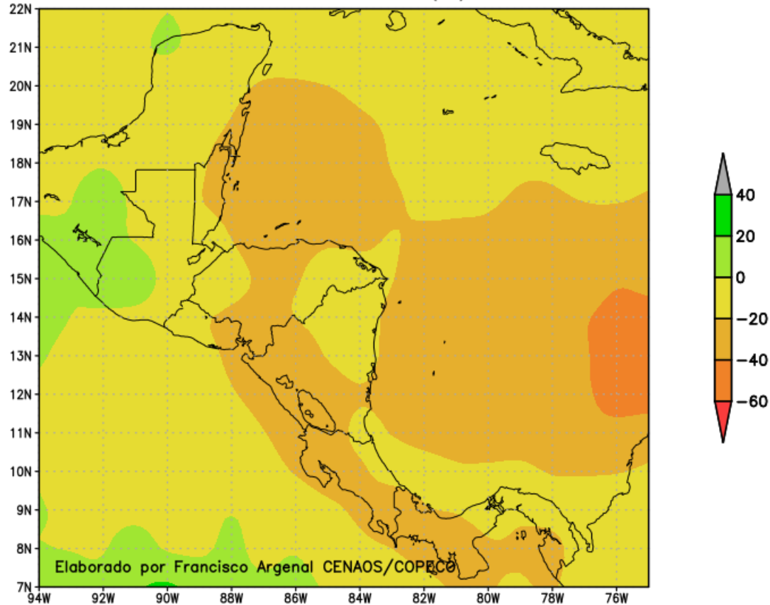
"Pronostico de anomalia de lluvia (%), Oct. 2026 NMME"
